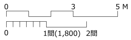
くにたち市民芸術小ホール 照明基本仕込み図 縮尺1/100
