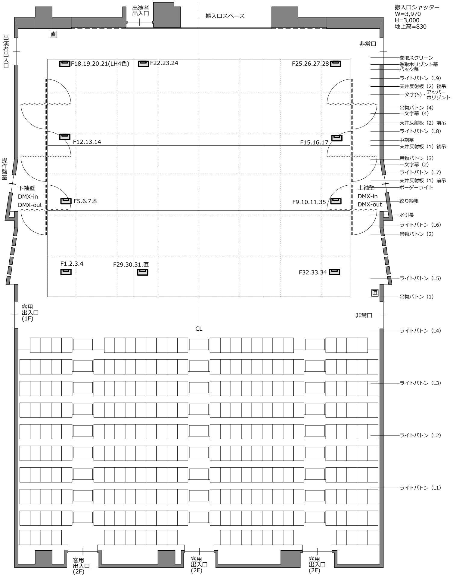
くにたち市民芸術小ホール 照明回路図(ステージ) 縮尺1/100
